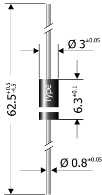
Dimensions - Maße [mm]
