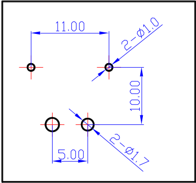
安装孔示意图
