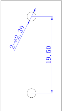
安装孔尺寸:
