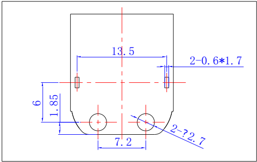
安装尺寸示意图
