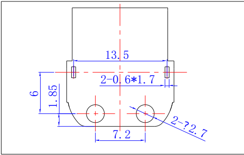
安装尺寸示意图
